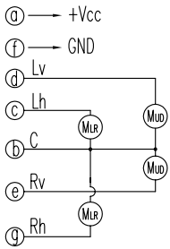
示意图 SCHEMATIC
