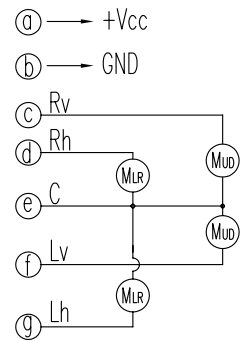
示意图 SCHEMATIC
