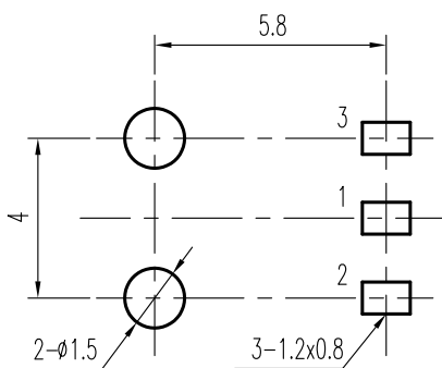
安装孔 PIERCING PLAN
