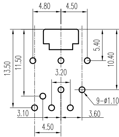
安装孔 PIERCING PLAN
