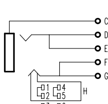
示意图 SCHEMATIC
