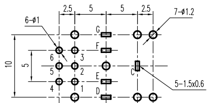
安装孔 PIERCING PLAN
