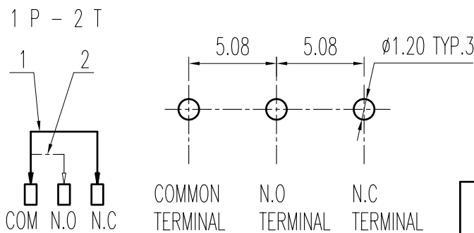
安装孔 PIERCING PLAN
