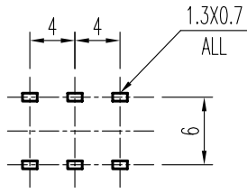
安装孔 PIERCING PLAN
