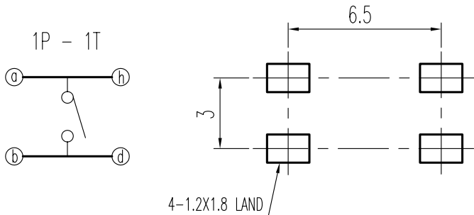
安装孔 PIERCING PLAN
