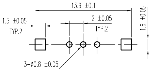
安装孔 PIERCING PLAN
