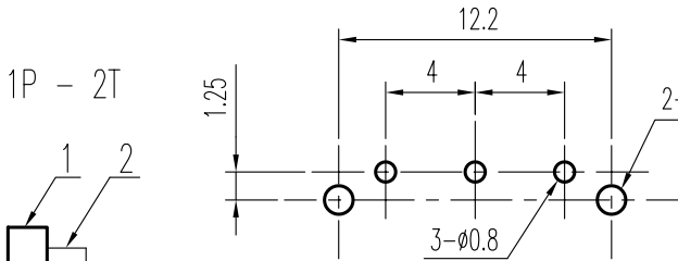
安装孔 PIERCING PLAN
