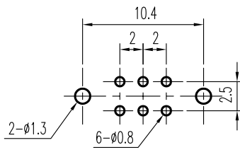
安装孔 PIERCING PLAN
