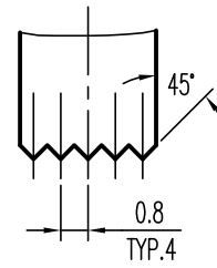
P DETAIL 5 : 1
