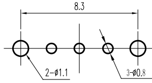
安装孔 PIERCING PLAN
