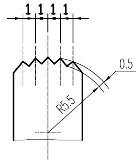
P DETAIL 2 : 1
