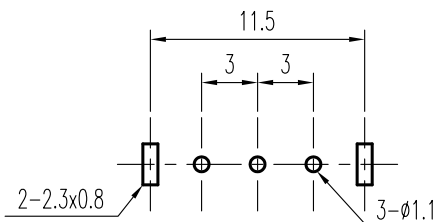
安装孔 PIERCING PLAN
