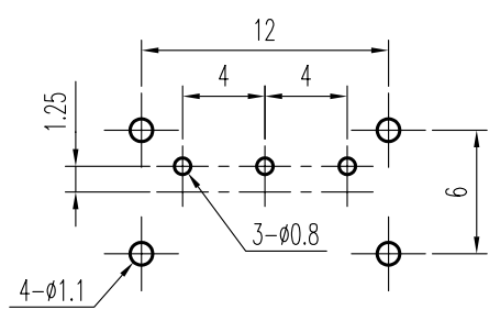
① 安装孔 PIERCING PLAN
