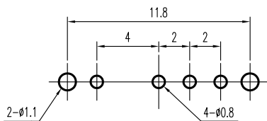
安装孔 PIERCING PLAN
