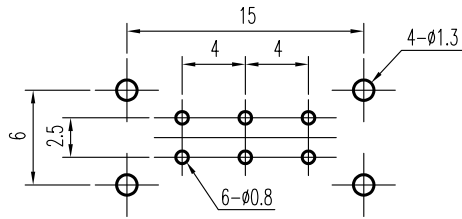
安装孔 PIERCING PLAN
